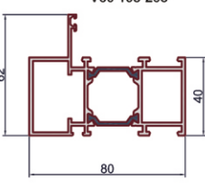
Усиленные профили
