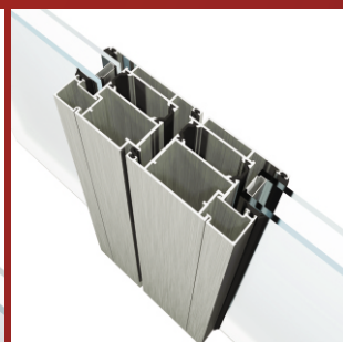
БЕЗШТУЛЬПОВОЙ ВАРИАНТ
