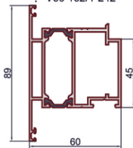
Импост
