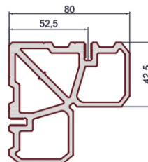
Сухарный профиль
