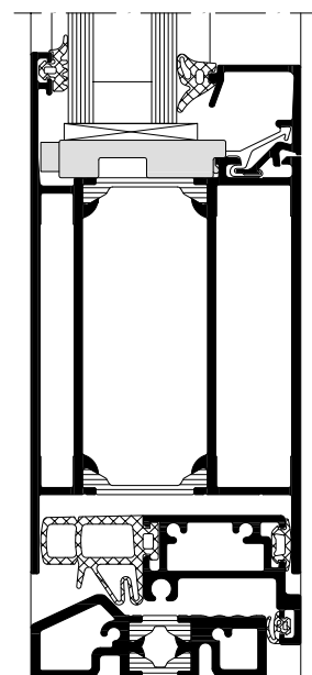
Schüco Дверь ADS 65, масштаб 1:2 Schüco Door ADS 65, scale 1:2
