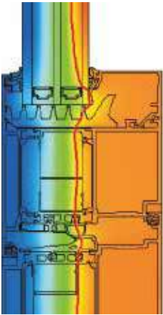
Прохождение изотерм Schüco ADS 90.SI Isothermal flow for Schüco ADS 90.SI
