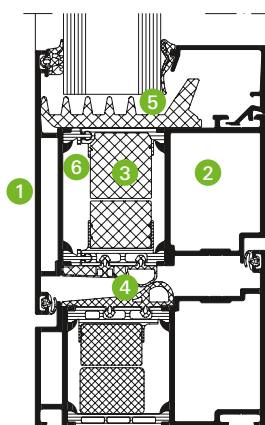
Schüco ADS 90.SI детальный вид, масштаб 1:3 Schüco ADS 90.SI in detail, scale 1:3
