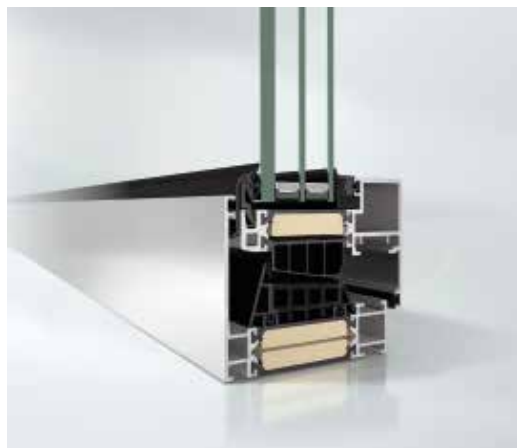
Schüco Окно AWS 90 BS.SI+ Schüco Window AWS 90 BS.SI+
