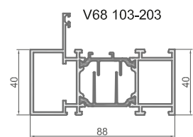
Усиленный профиль с одним усом
