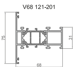
Импост узкий
