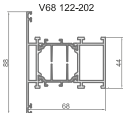
Импост широкий
