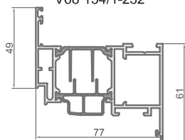
Створка широкая "прямая"
