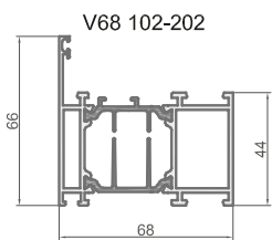
Рама широкая
