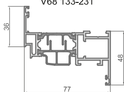
Створка узкая "прямая"
