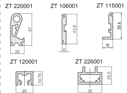
Вкладыши и дополнительный профиль
