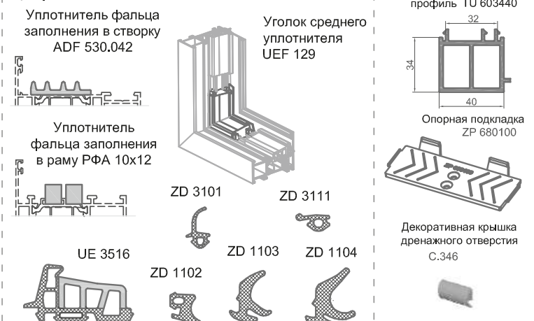
Профили из ЭРДМ и вспененного полистирола
