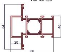
Усиленные профили
