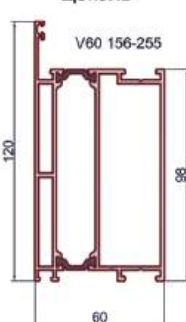
Цоколь
