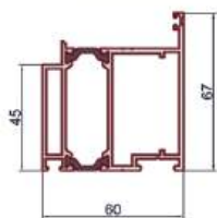
Рама внутреннего открывания
