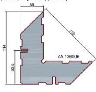
Вкладыши (штучная деталь)
