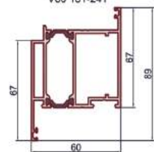
Штульп внутреннего открывания
