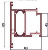
Створка внутреннего открывания
