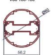
Поворотный профиль
