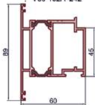
Импост
