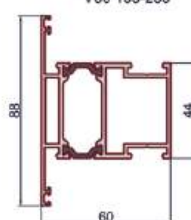
Порог
