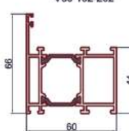
Цоколь
