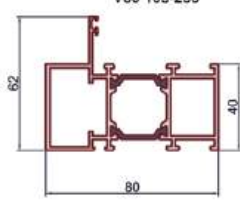
Усиленные профили
