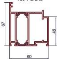
Штульп наружного открывания
